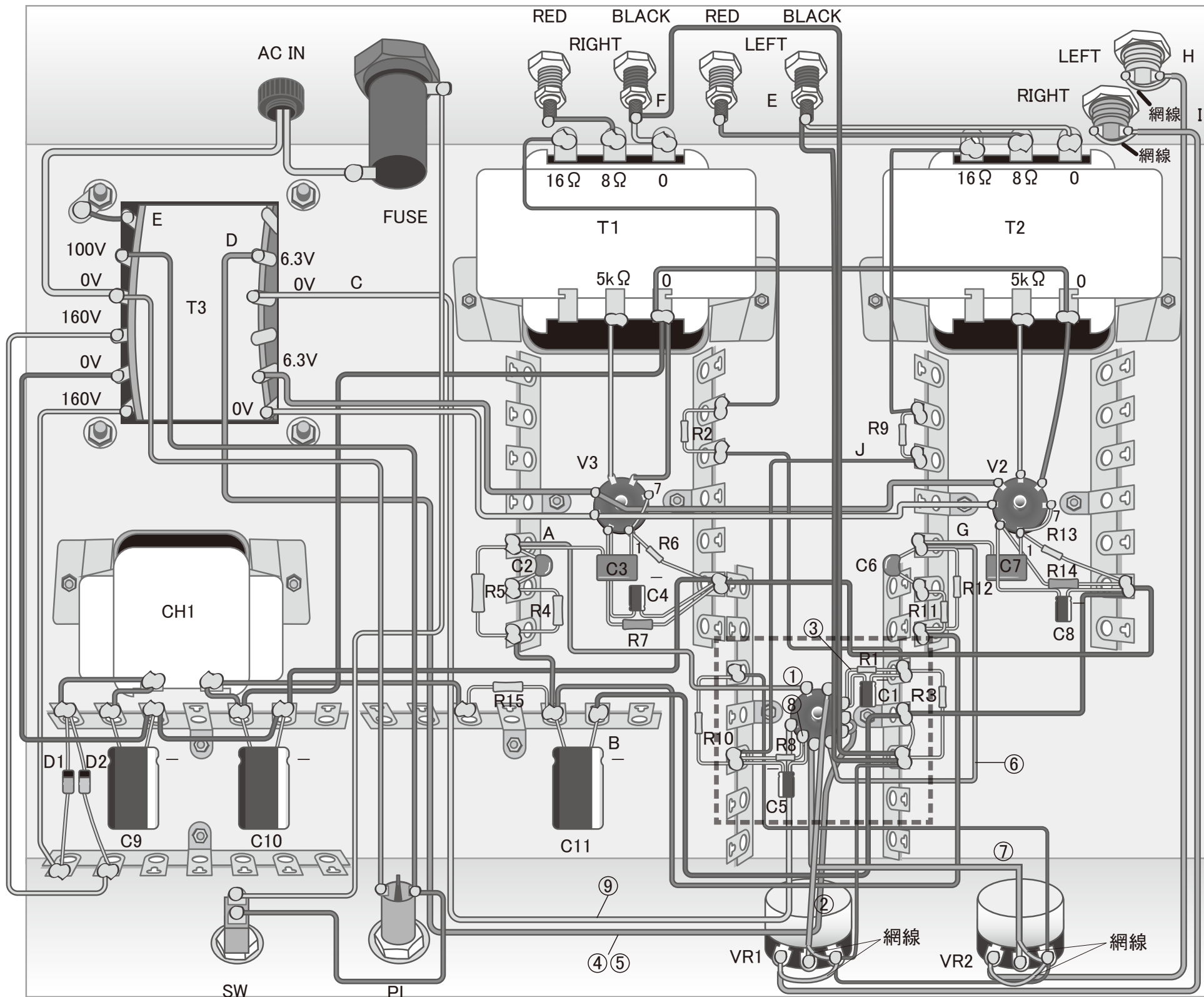
実体配線図
