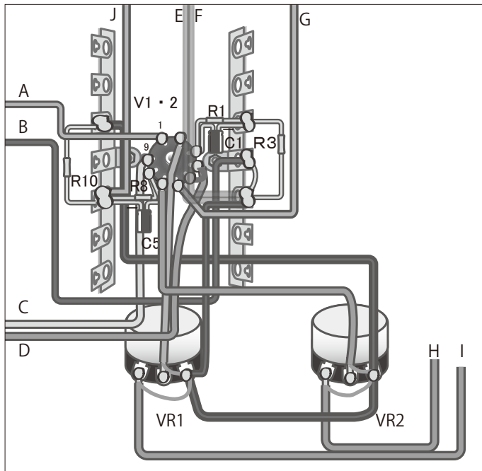
12AX7 (V1・2) 部分拡大配線図 (見やすくするためこの拡大図では一部の配線を省略しています)
